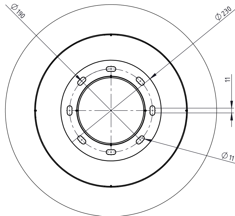
SZCZEGÓŁ D SKALA 1 : 5
